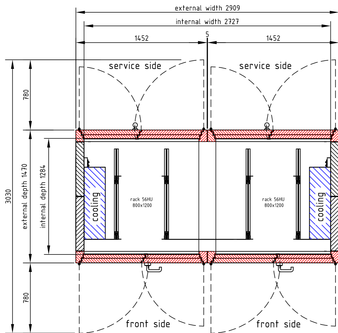
A-A ( 1 : 25 )
