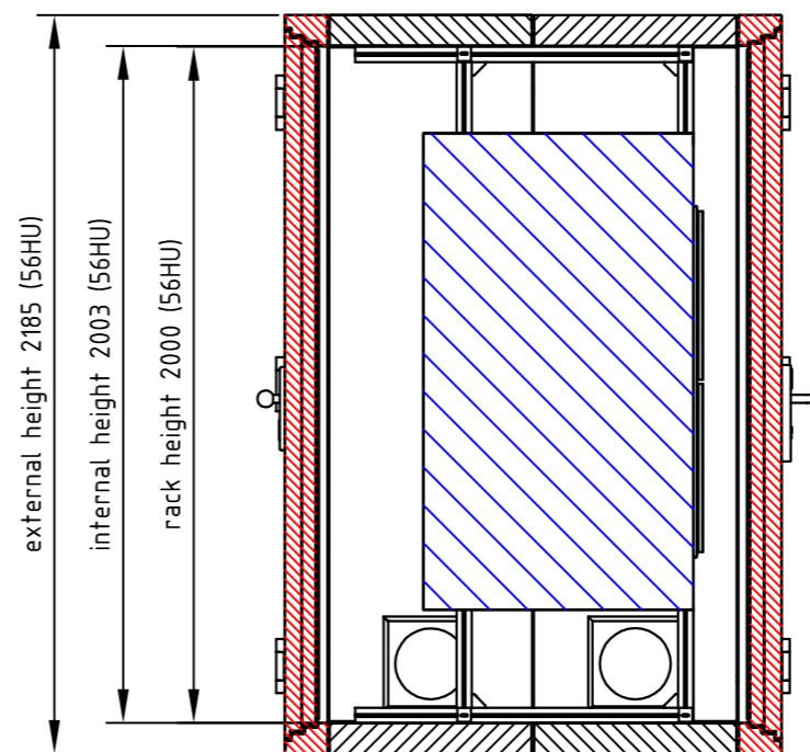
B-B ( 1 : 25 )
